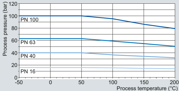
Metric flange ratings, EN 1092-1
